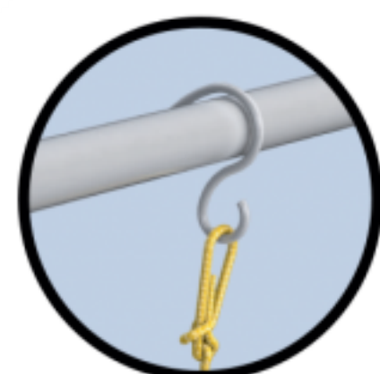
HookIT
