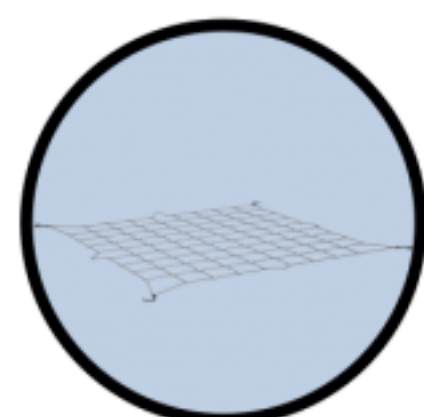
WebIT
